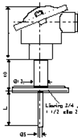
P2209 med inbyggd transmitter
