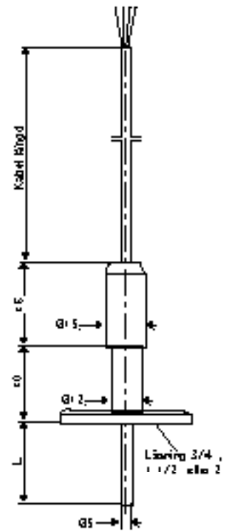
P2209 med PTFE kabel
