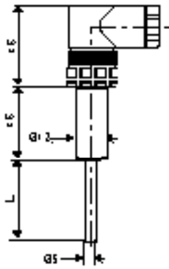
P2209 med EC 947-5-2 kontakt
